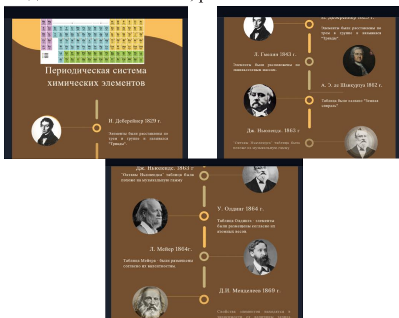
Рис.2. Фрагмент таймлайна по истории создания периодической системы химических элементов
