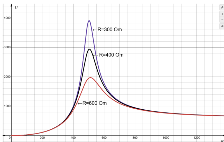
6-расм. Резонанс эгри чизиклари
